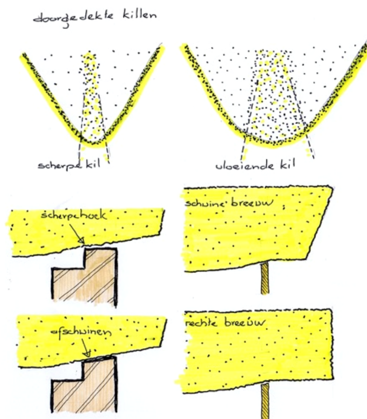
Figuur 3: Voorbeelden van een scherpe kil en een vloeiende kil. Detailering van een (streekgebonden) rechte of schuine breeuw.
